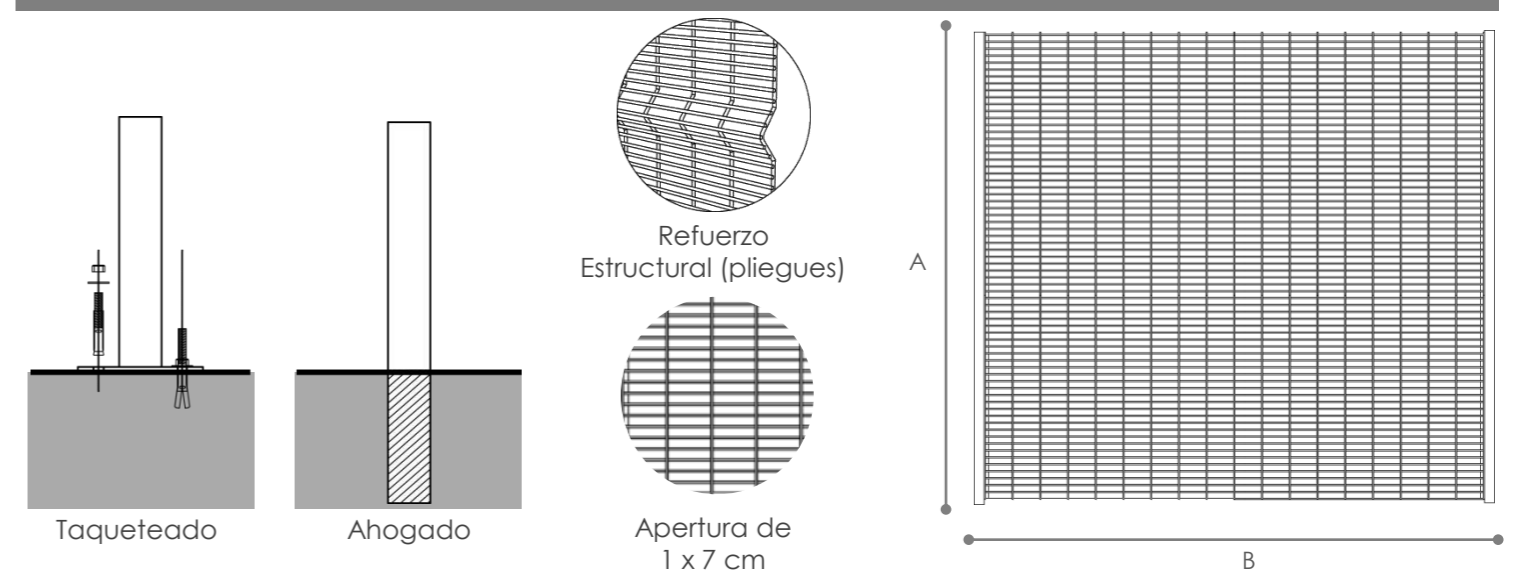
ANCLAJE
