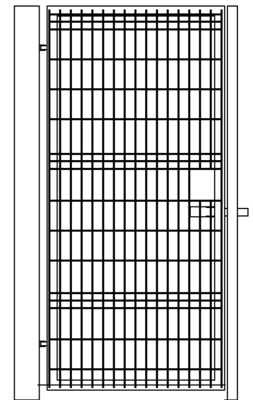
PUERTA PEATONAL
