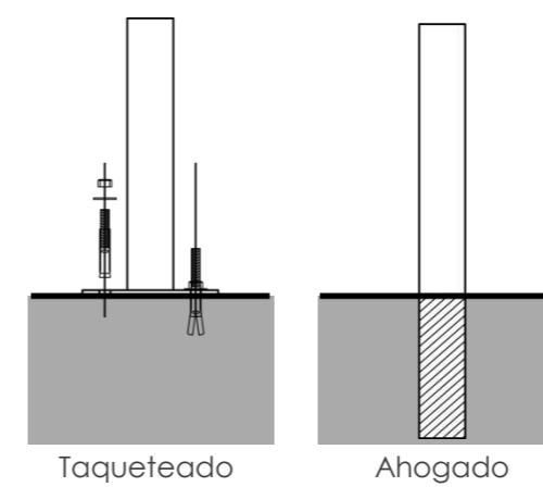
ANCLAJE
