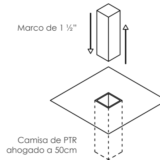
ANCLAJE
