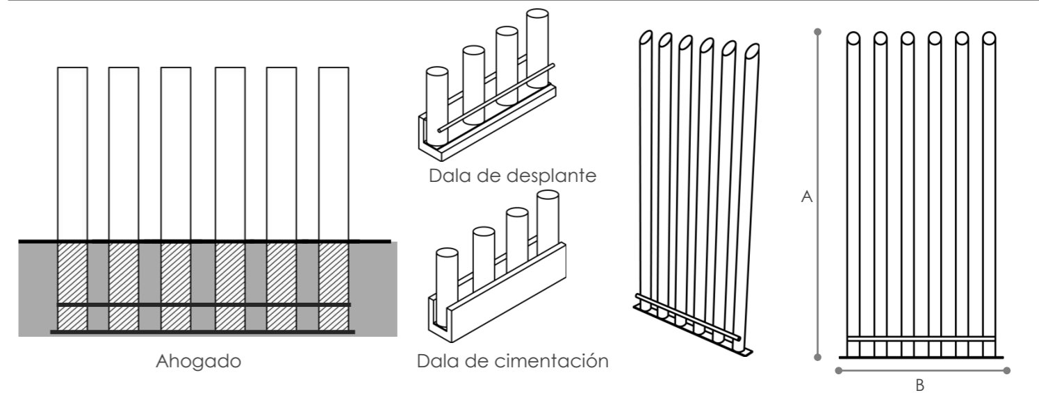
ANCLAJE
