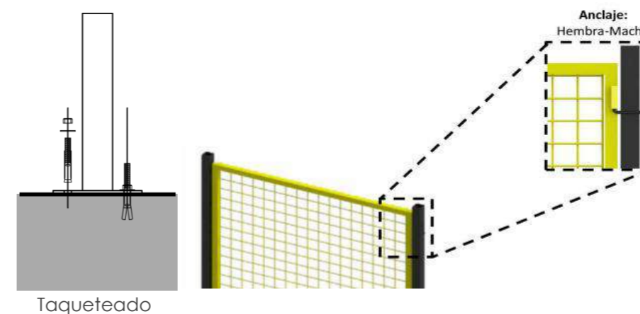
ANCLAJE
