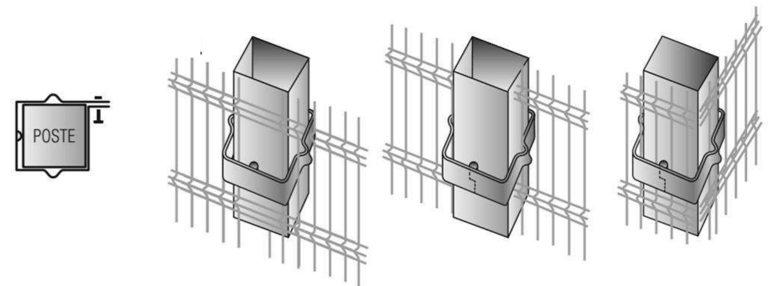
SUJECIÓN DE CERCA CON ABRAZADERAS CERCASEL
