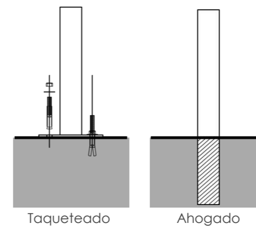
ANCLAJE
