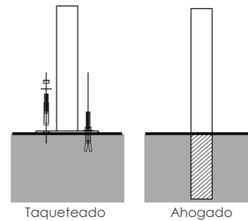
ANCLAJE
