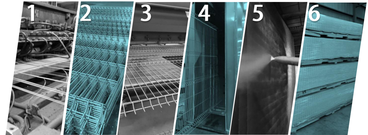
1 Electrosoldado 2 Corte a medida 3 Pliegues 4 Lavado y secado 5 Pintura electrostática 6 Terminado
